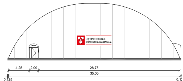
ANSICHT OSTEN
